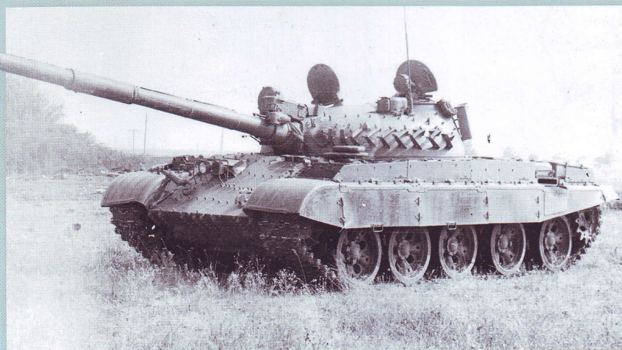
★ Средний танк Т-62МВ. На башне и корпусе хорошо видны бонки и кронштейны для крепления элементов комплекса динамической защиты.
